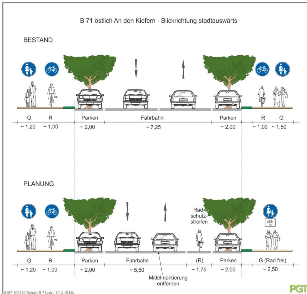
Abb. 6.2: Beispiel: Querschnitt B 71 - Markierung eines einseitigen Radschutzstreifens
